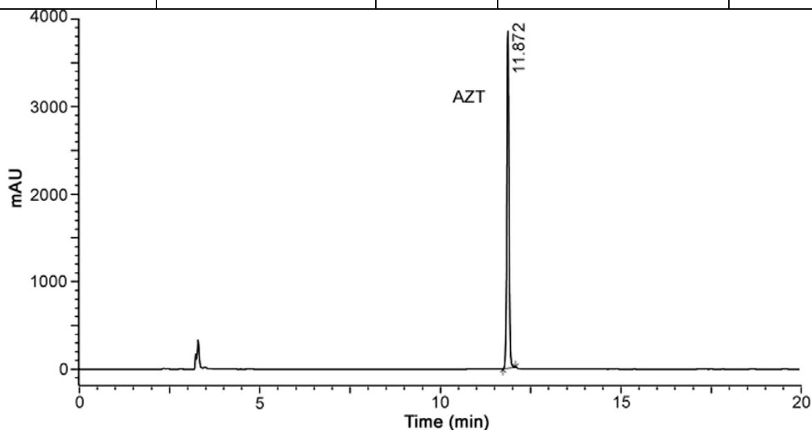
Fig. 1. Chromatogram of AZT (2 mg/mL).
